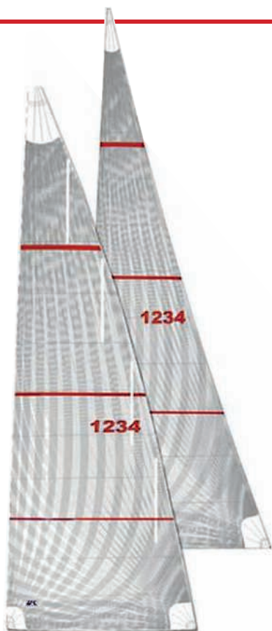
UK X-Drive® Max Roach Rollgroßsegel mit und ohne vertikale Rundlatten
